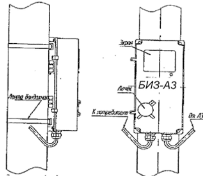
Вариант установки БИЗ-А3 на столбе с помощью стальной бандажной ленты
